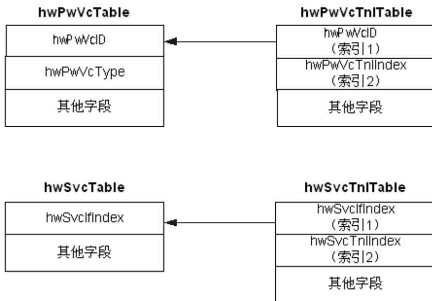
图 104-1 VC 配置表和 VC 隧道信息表的关系
